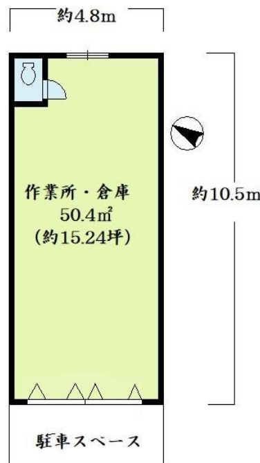
【間取図】
